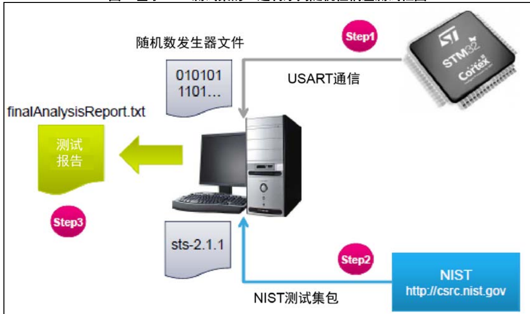
图2. 基于NIST测试集的二进制序列随机性偏差测试框图
