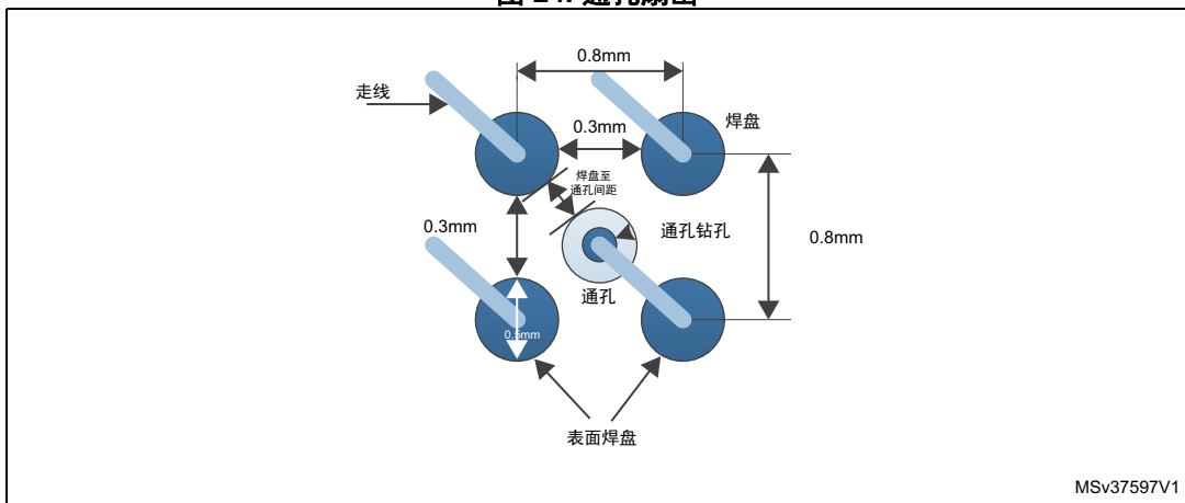
图 25. FMC 信号扇出布线实例
