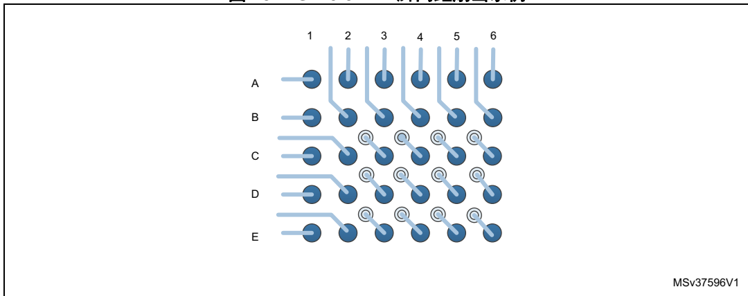
图 24. 通孔扇出
