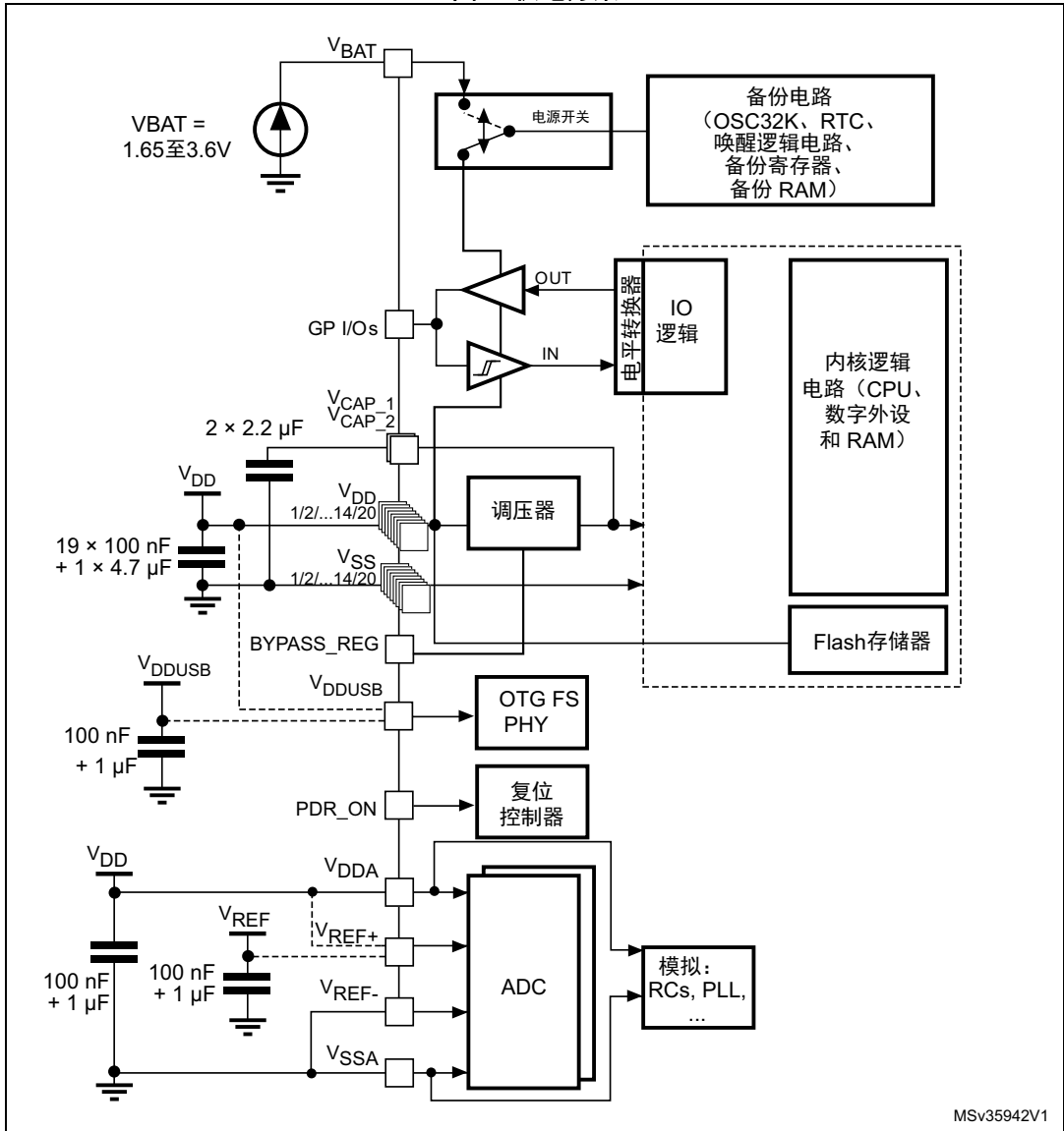
图 3. 供电方案
