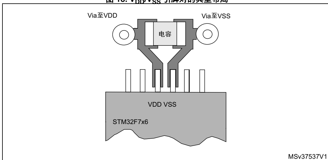
图 18. V DD /V SS 引脚对的典型布局
