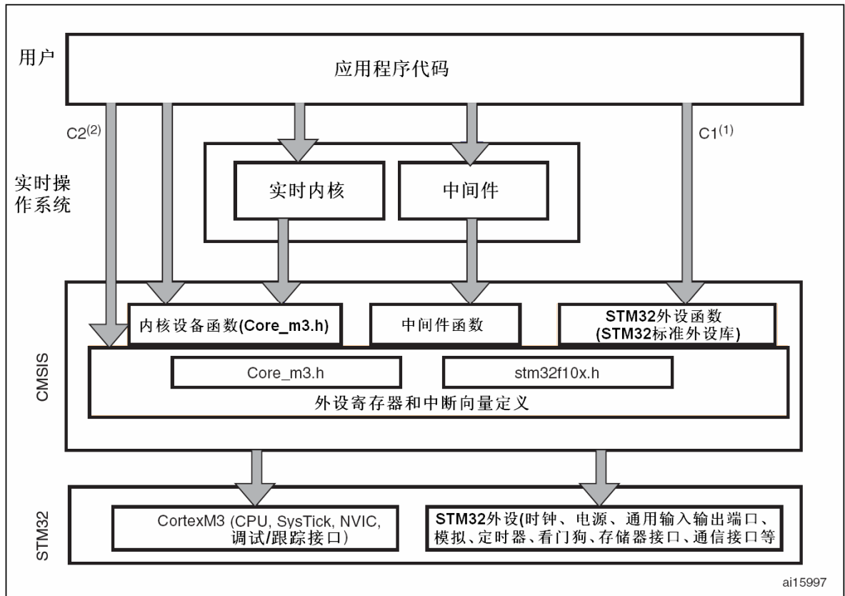
图5 STM32库和CMSIS：结构
