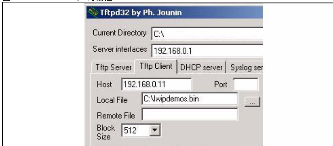
图 4. TFTPD32 对话框
