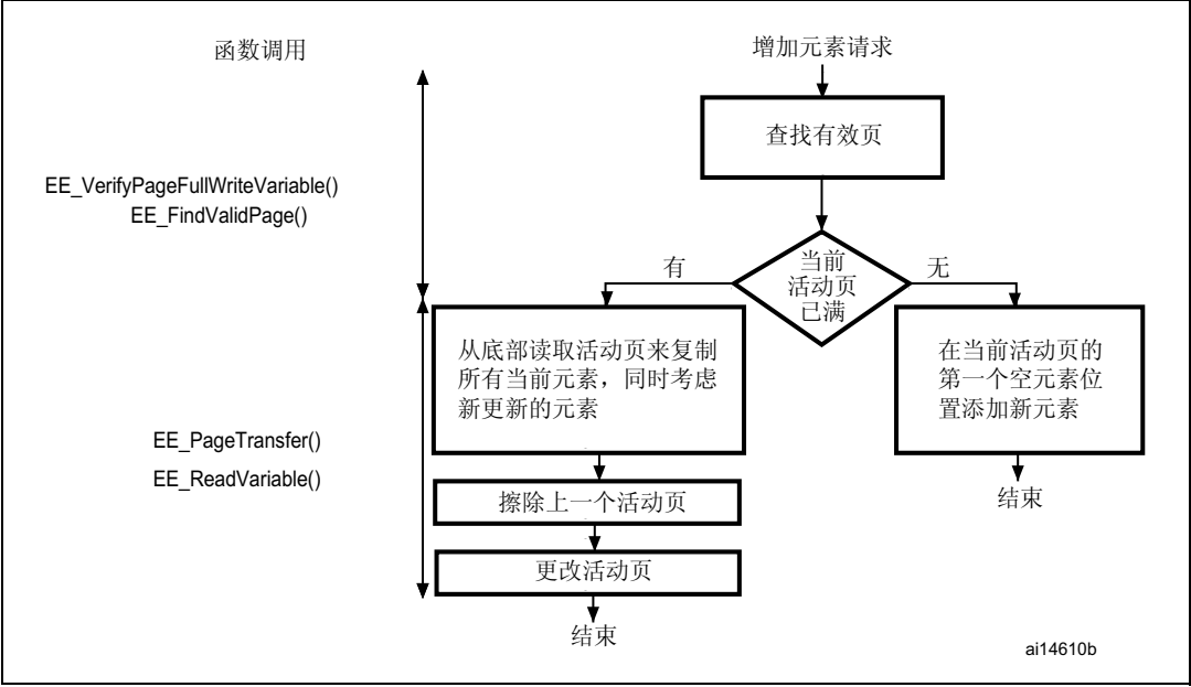
图 4. WriteVariable 流程图
