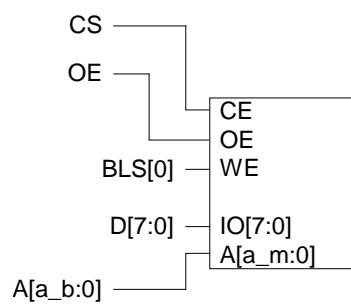
图 5.23 16 位存储器组的外部存储器接口
