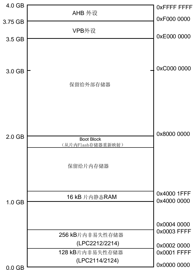
图 5.5 系统存储器映射
