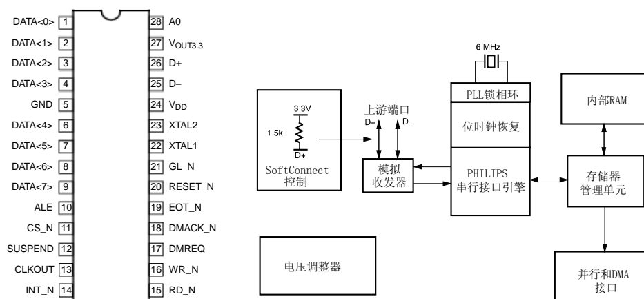
图 6.70 PDIUSB12 管脚排列及内部功能框图
