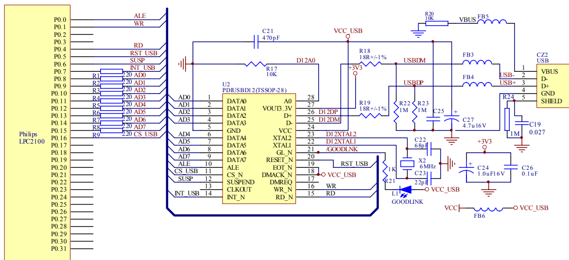
图 6.72 LPC2100 与 PDIUSBD12 连接电路图
