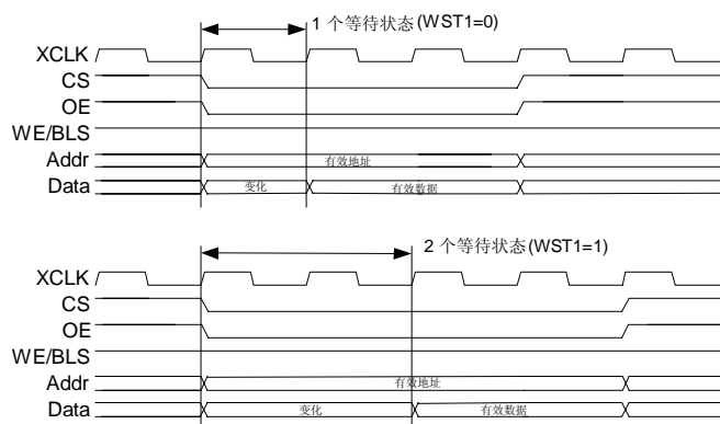
图 5.25 外部存储器读访问 (WST1=0 和 WST1=1 两种情况)
